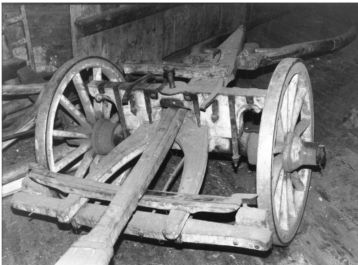
17. Parte anteriore del carro (bròzo davànte)
