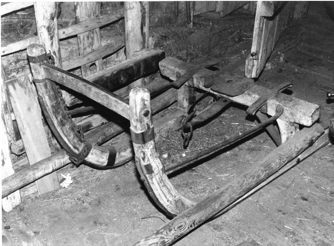
19. Slitòn: Slitta da carico in legno
