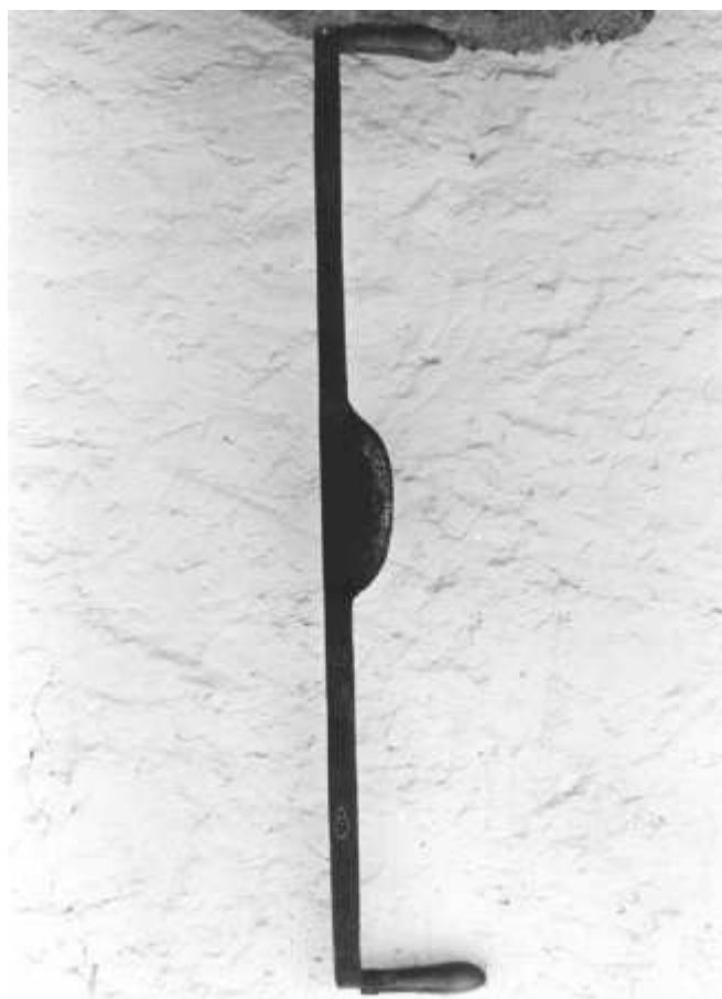
3. Fèr a dóe man: serviva a smussare la testa dei tronchi
